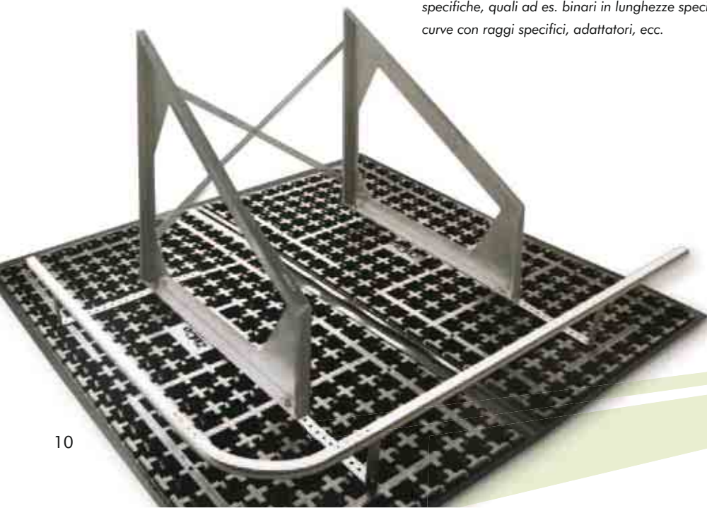
La protezione anticaduta può essere facilmente combinata con la struttura di sostegno ZinCo grazie al sistema modulare.
