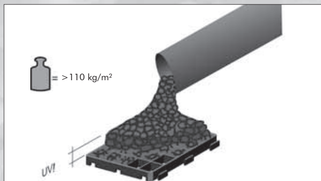
6. Apporto della zavorra necessaria (al min. 110 kg/m 2 )
