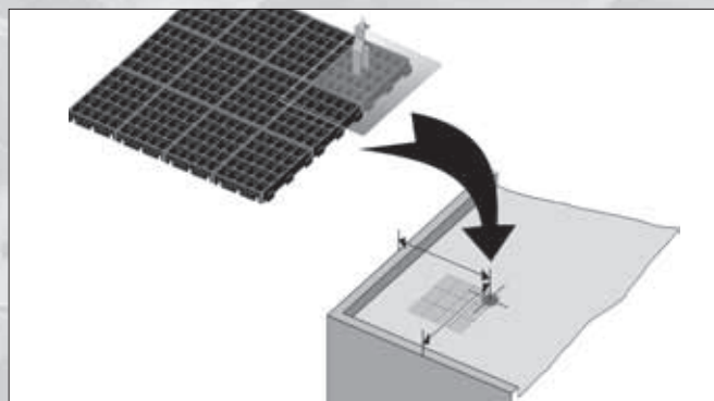
4. Posizionamento del gruppo di griglie incluso il punto di ancoraggio
