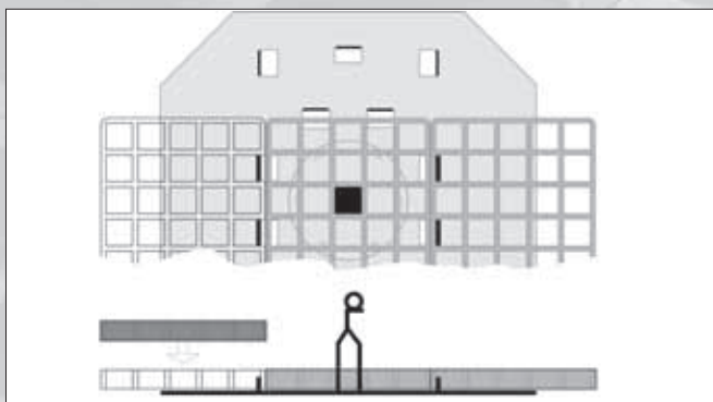
3. Le griglie devono essere poggiate uniformemente sulla piastra di base e le linguette verticali devono incastrarsi negli elementi vicini.
