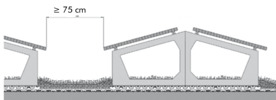
Montaggio solare a "due falde"
