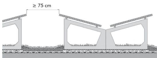
Montaggio solare a "farfalla"
